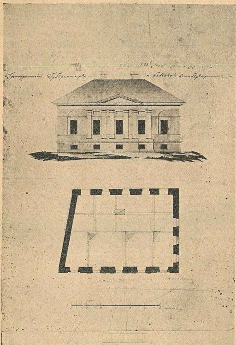
Підписаний кресленик архітекта Ярославського р. 1801, інв. МУМХ № 5373.
