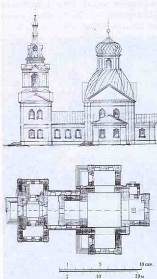
Рис. 43. Креслення Георгіївської церкви с. Ковчина.
