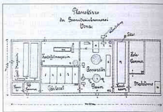
План-схема гуральні у колонії Окна, що належала Вікторії Ранді. 1923 рік
